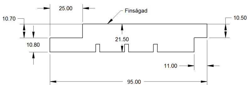
Nr. 540 Falsad spårpanel raka kanter 22x95
