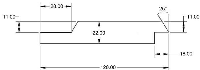
Nr. 201 Falsad spårpanel dubbelfas 22x120 VB2322
